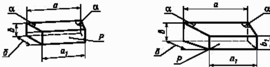
Рисунок 3 — Трапецидальный клин
